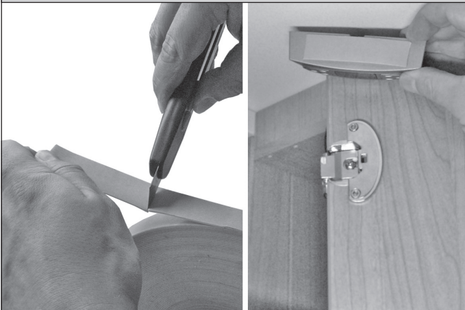
6. Beispiel: Anbringung der Sat-Maus / example: fixing Sat-Mouse / exemple ajouter la Sat-souris
